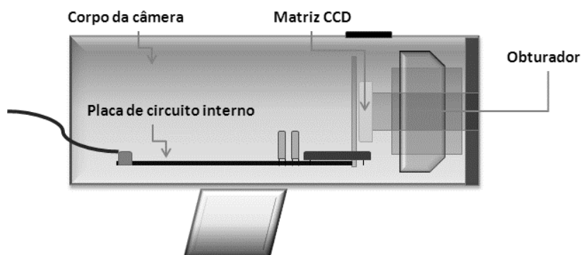
Figura 1.15 – Representação esquemática de uma webcam . Adaptado de Almeida, 2012.
