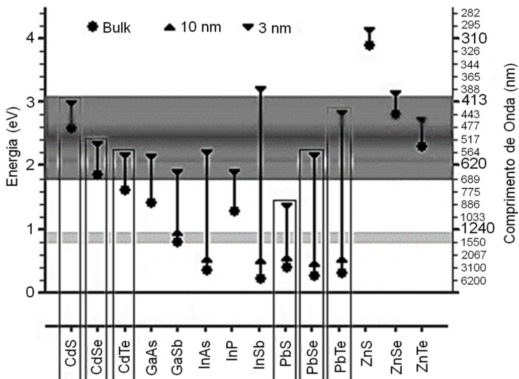
Figura 1.11. Representação esquemática para o controle das propriedades ópticas em PQs. Os PQs destacados correspondem as famílias de maior interesse do grupo, as de bandgap sintonizável no visível (CdS, CdSe e CdTe) e na região das comunicações ópticas (PbS, PbSe e PbTe). Ilustração adaptada de Moreira, 2005.
