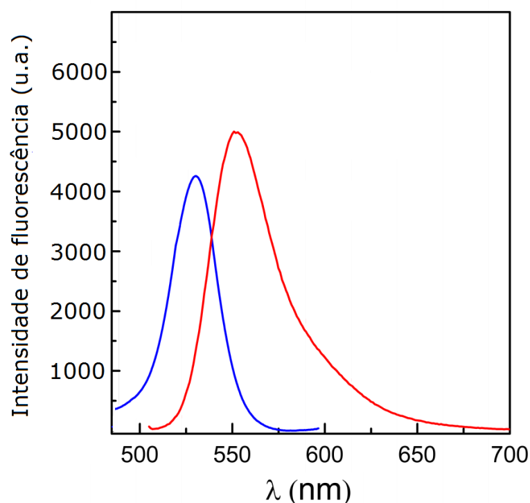
Fig. 3.4 – Representação de espectro de emissão fluorescente para padrão de rodamina 6G (linha vermelha) e nanocristais de CdTe (linha azul).
