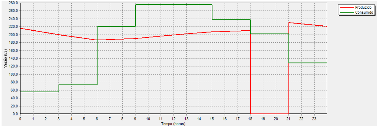
Figura 30 - Balanço de vazão do Cenário 8 do sistema com parada de bombeamento no horário de ponta.
