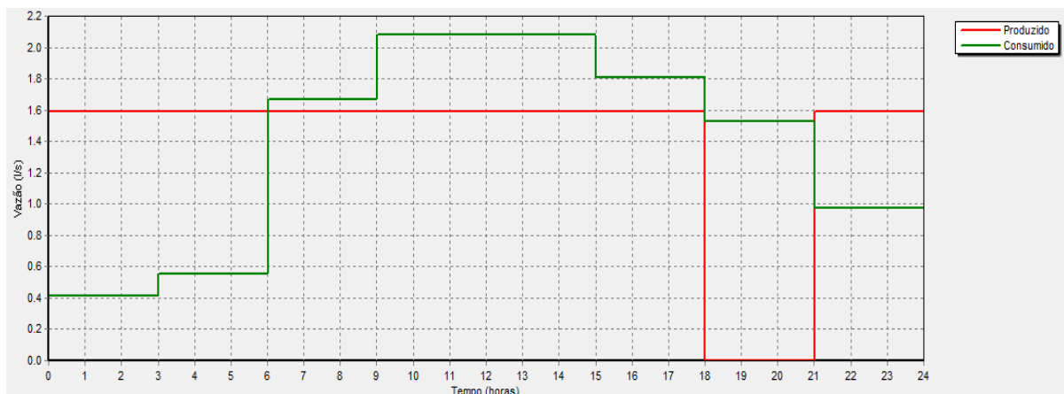
Figura 27 - Balanço de vazão da edificação com 20 pavimentos com parada de bombeamento.
