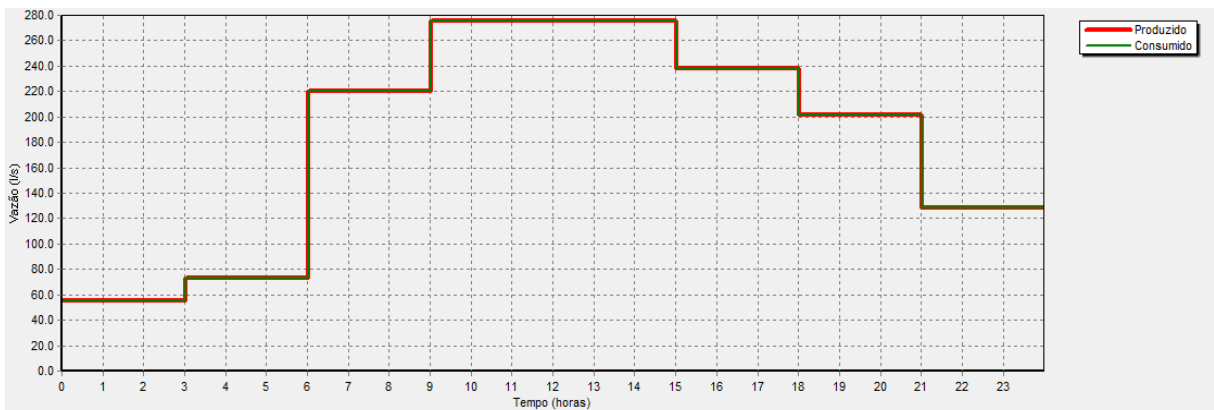
Figura 31 - Balanço de vazão do Cenário 8 do sistema com bombeamento direto.
