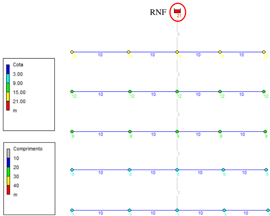
Figura 4 - Modelagem de edifício com 5 pavimentos do sistema com pressão mínima na entrada de 10 mca.
