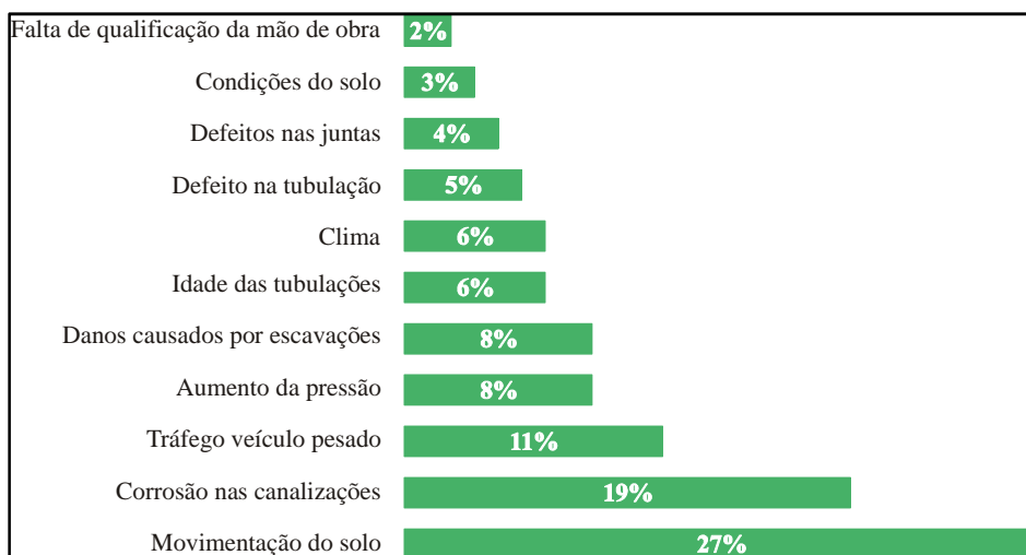
Figura 2.3 – Fatores que influenciam o aumento das perdas reais
