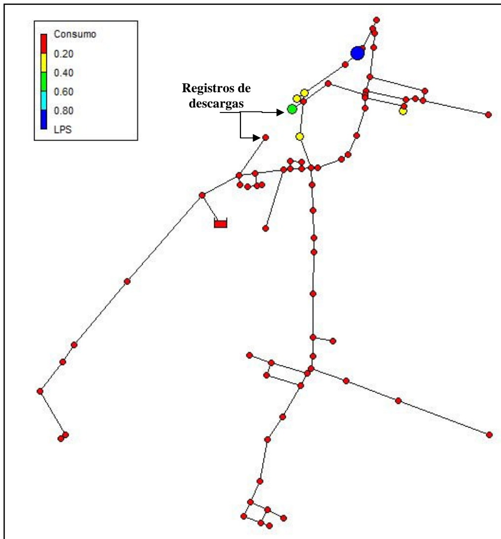
Figura 5.29 – Estimativa dos consumos após a calibração, utilizando os parâmetros vazão e rugosidade das tubulações
