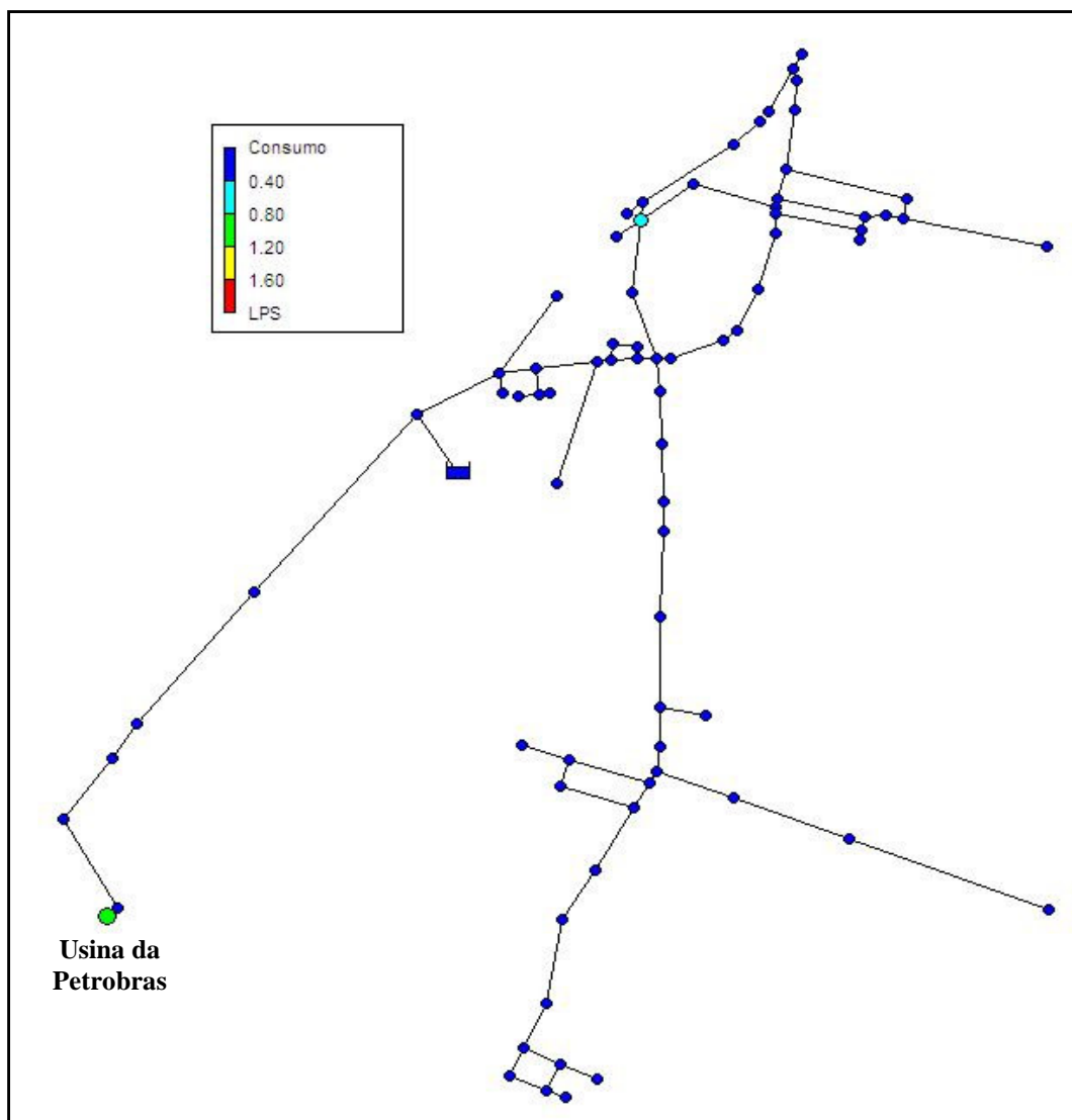
Figura 5.27 – Estimava de consumo após a calibração, utilizando o parâmetro vazão
