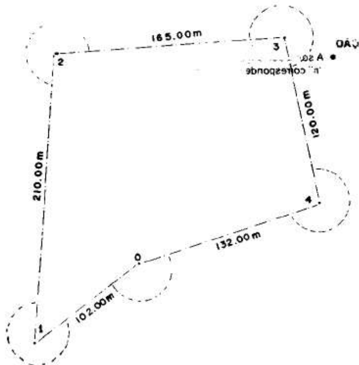
Fig. 1: Caminhamento com ângulos internos.
