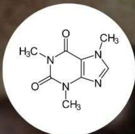
Estrutura química da cafeína
