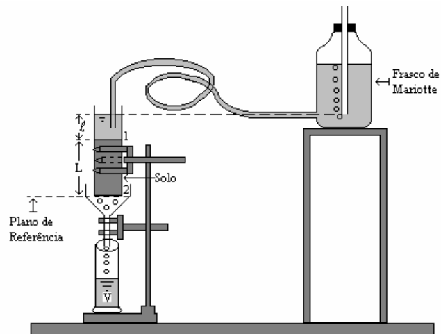
Figura 13. Esquema de um permeômetro de coluna vertical e carga constante (Ferreira, 2002).
