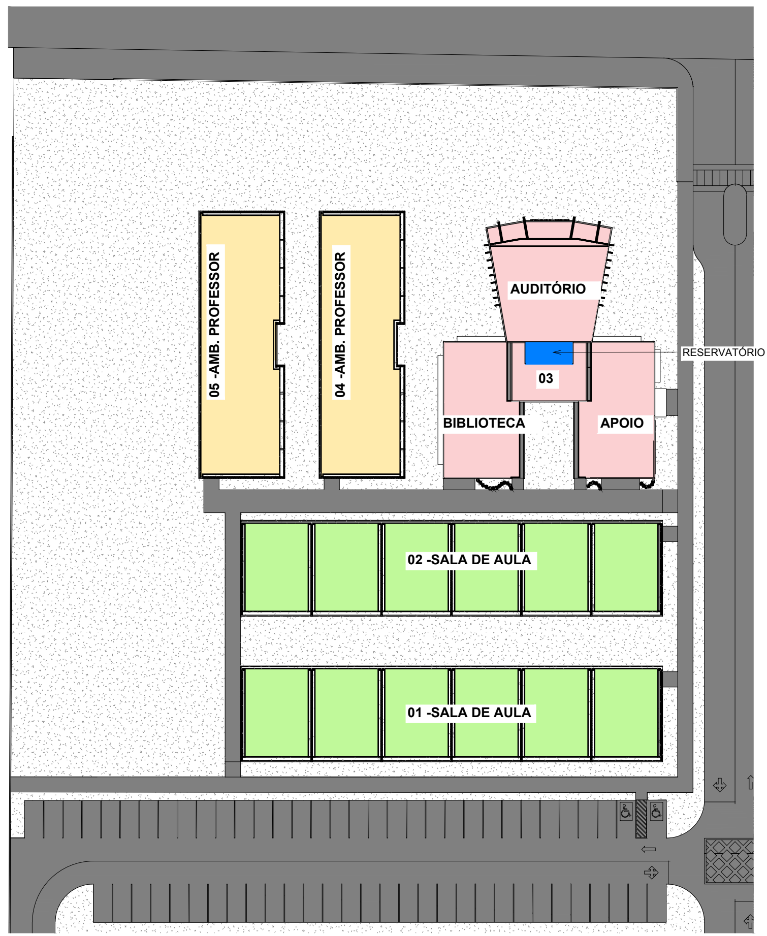
3 PLANTA DE LOCALIZAÇÃO - SANTA RITA ESCALA 1/500
